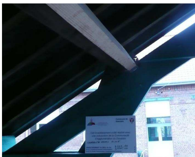
Réhabilitation de la charpente du préau de l'école Mireille du Nord.
